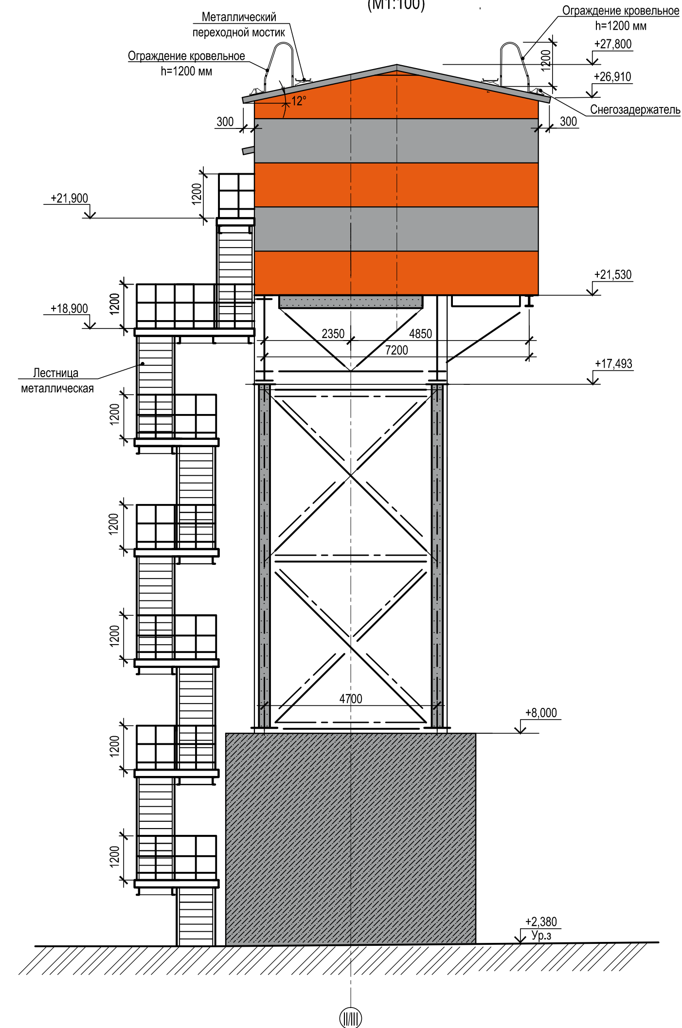
Фасад I/III (М1:100)
