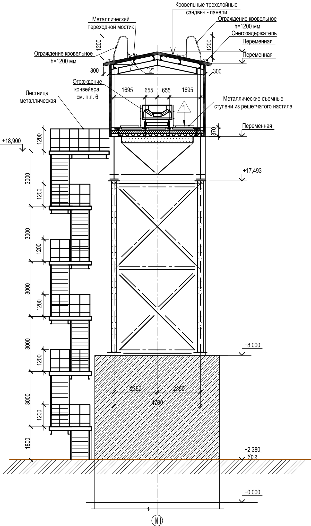
Разрез 2-2
