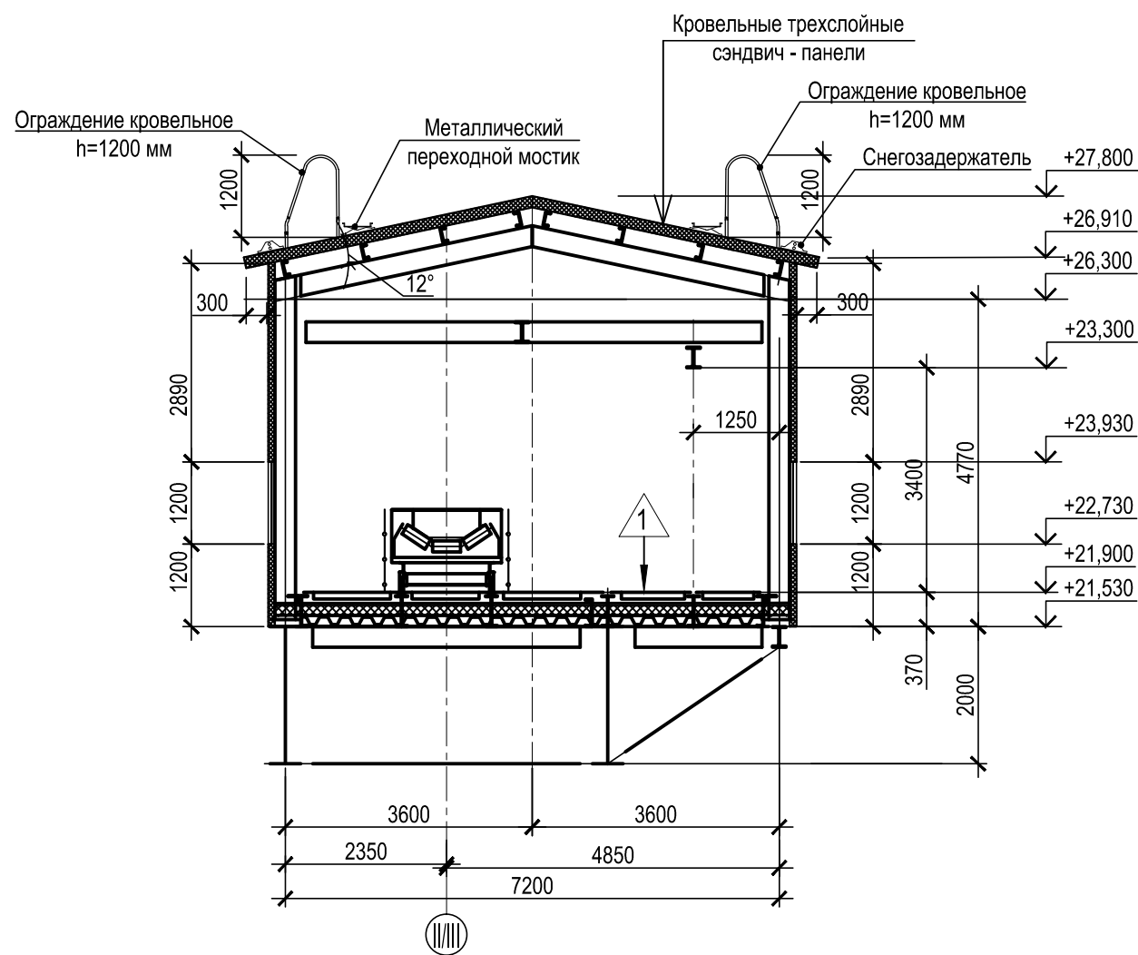
Разрез 3-3
